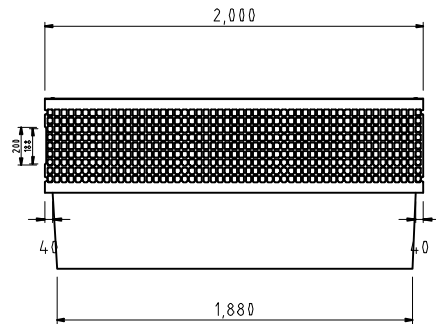
消音型可変側溝 スタンダード・土留付 蓋付
