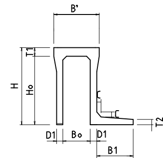
消音型可変側溝 スタンダード土留付 蓋付
